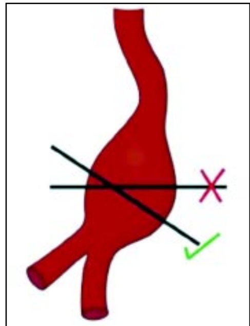
Figura 2. Medición de saco aneurismático. Diagrama que representa la correcta (positivo verde) e incorrecta (equis roja) medición del saco aneurismático en una aorta tortuosa. Las mediciones oblicuas incorrectas sobreestiman su diámetro.
